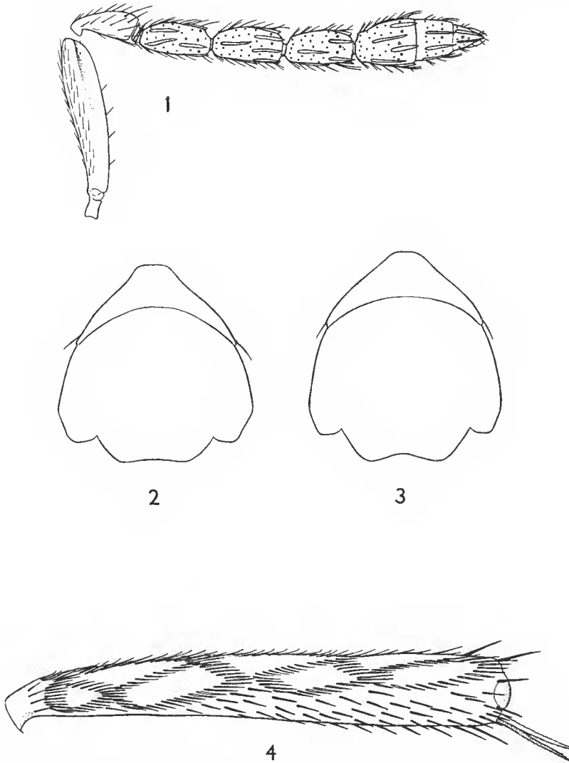
FIGS 1-4. — Elasmus species : 1, E. maderae sp. n., ♀, right antenna ; 2, E. maderae , ♀, pronotum and mesoscutum ; 3, E. steffani Viggiani, ♀, pronotum and mesoscutum ; 4, E. maderae sp. n., ♀, left hind tibia.
